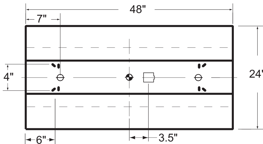
DUAL PENDANT
